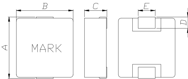
Dimension (Unit:mm)
