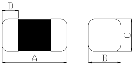
Dimension (Unit:mm)
